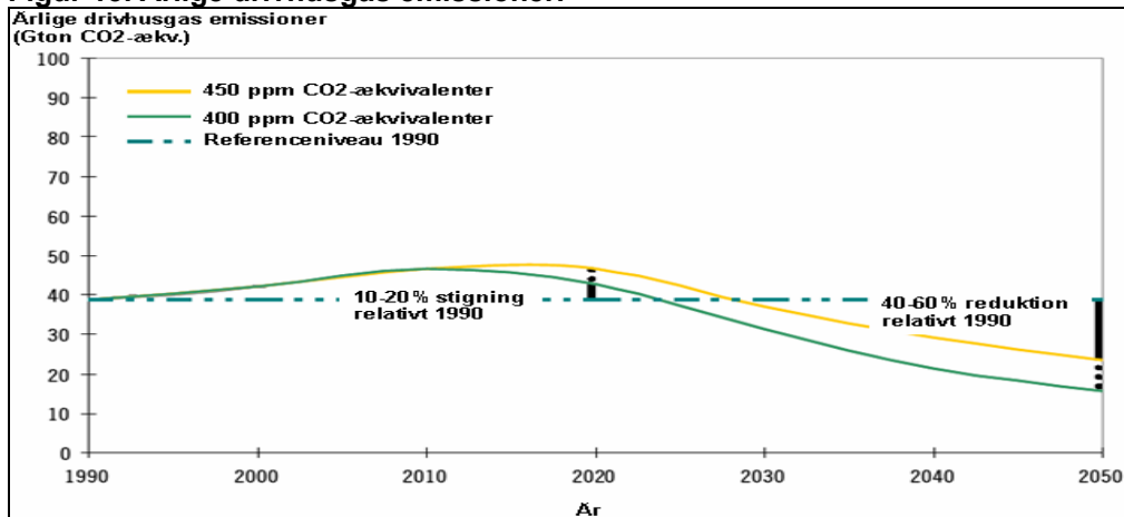
Figur 13. Årlige drivhusgas emissioner.
