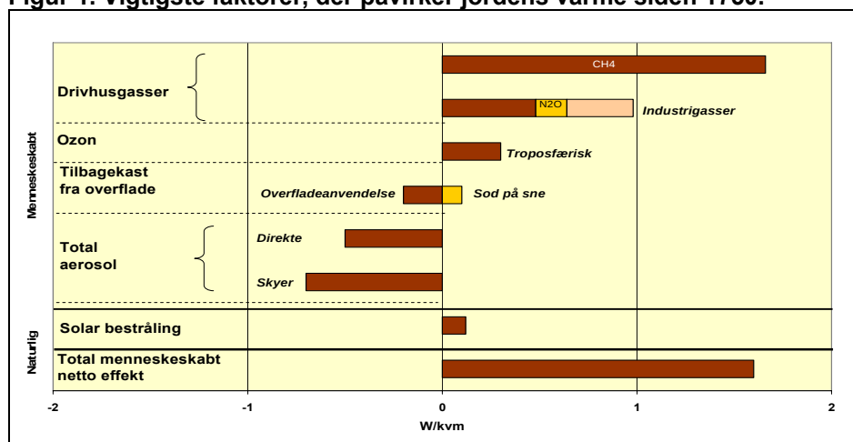
Figur 1. Vigtigste faktorer, der påvirker jordens varme siden 1750.
